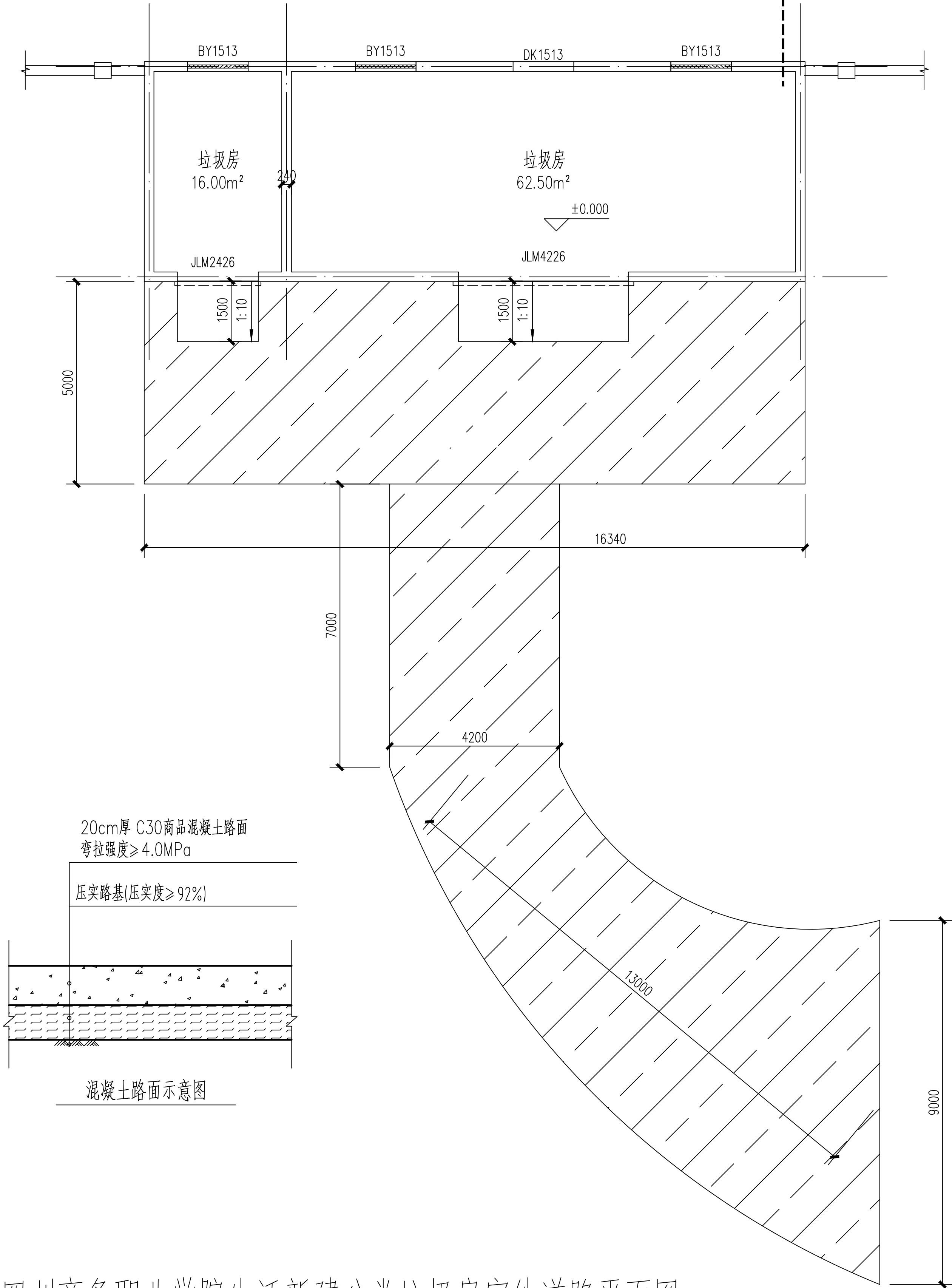
四川商务职业学院生活新建分类垃圾房室外道路平面图
